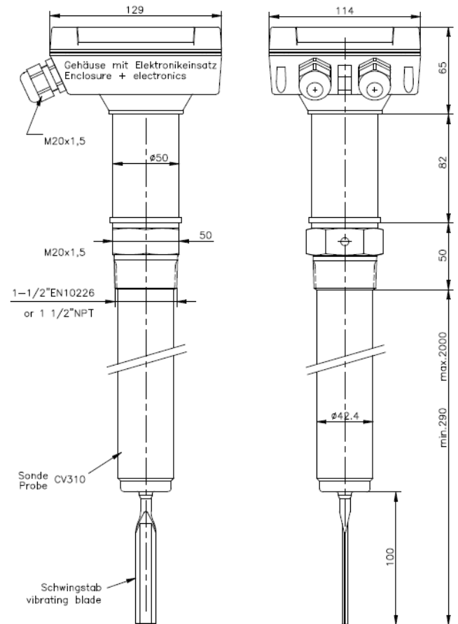
Sondermodell HT mit Temperaturisolierzwischenstück
